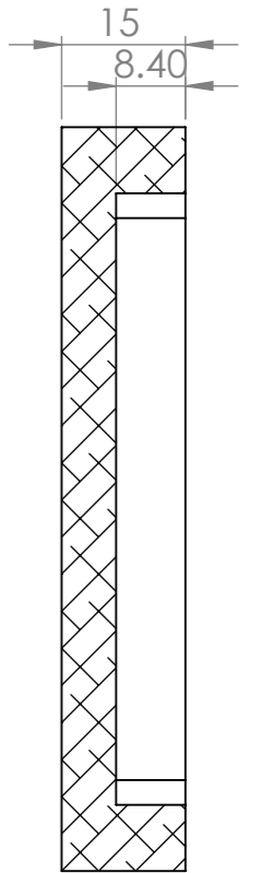
SECTION A-A
